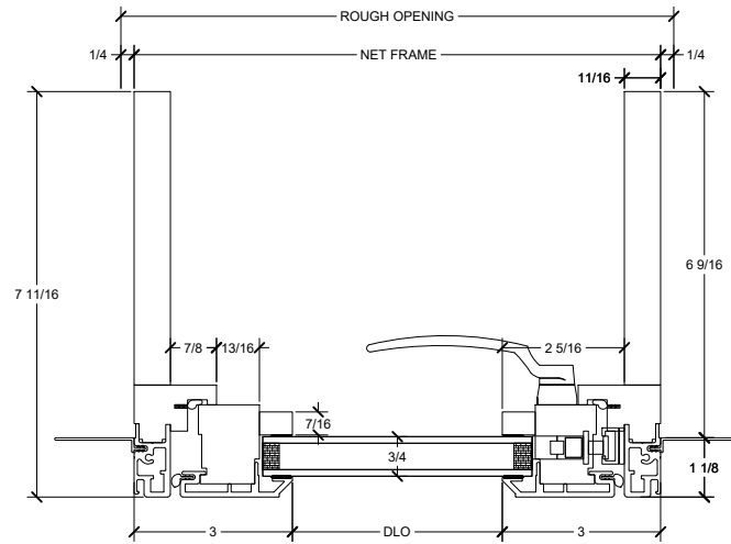
Jambs
