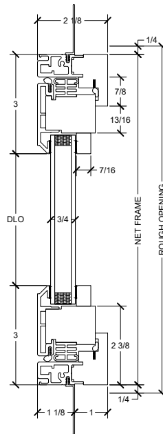
Head Jamb & Sill
