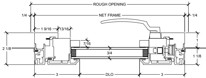
Jambs
