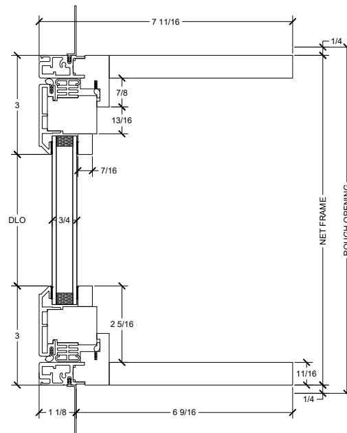
Head Jamb & Sill
