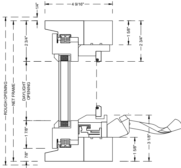
Head Jamb & Sill
